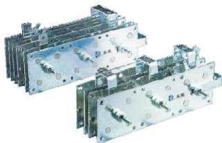
Rectifier Bridge
